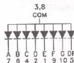
Anode Common(MD-5217)
