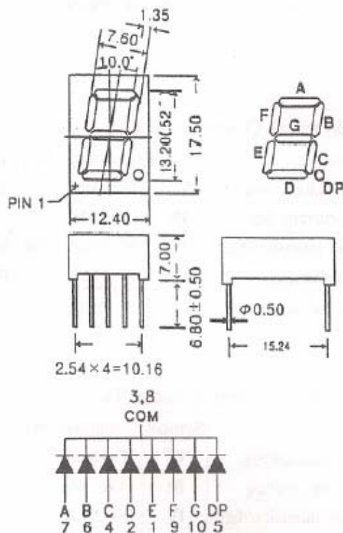
Cathode Common(MD-5210)
